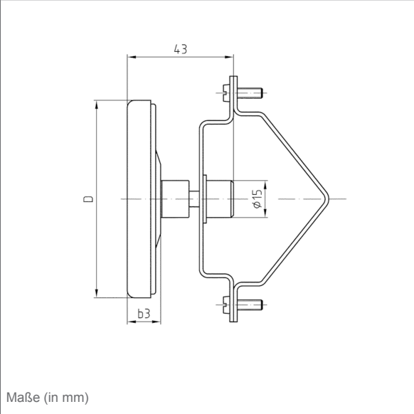
Anschluss axial, mit Universalschelle für Rohre 3/4" bis 1 1/2"
