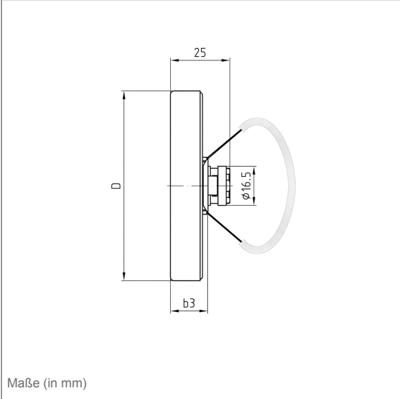
Anschluss axial, mit Befestigungsfedern
