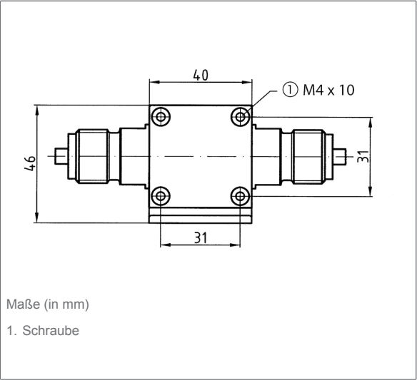
DMU 11 D - Anschluss 2 x G1/2B (EN 837)
