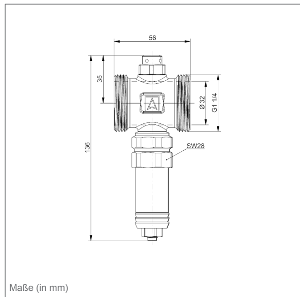
Frostschutzventil AAV 302
