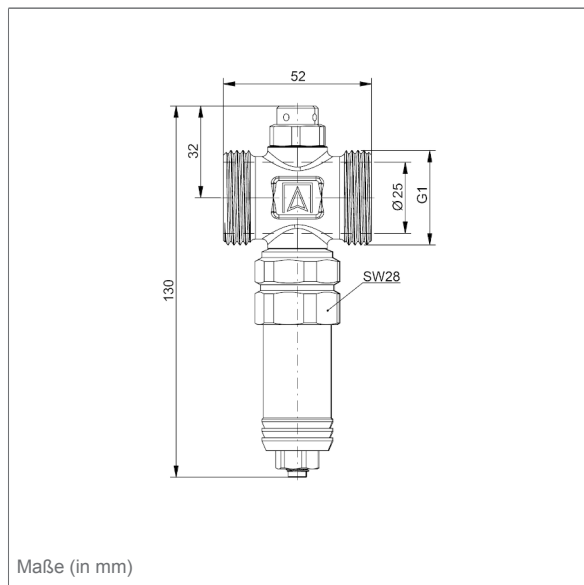
Frostschutzventil AAV 102
